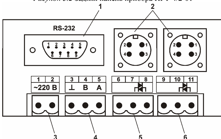
Рисунок 3.3 Задняя панель прибора ИРТ-4/2-02
