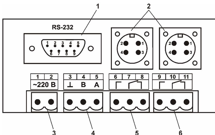
Рисунок 3.2 Задняя панель прибора ИРТ-4/2-01
