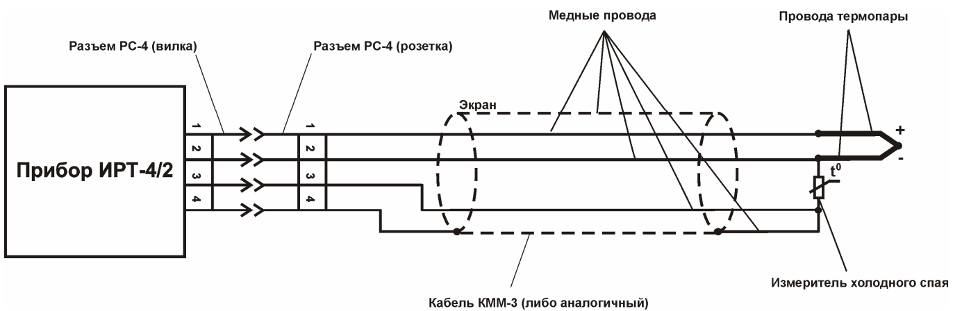
Рисунок 3.7 Схема подключения ТЭ преобразователей удлиненными медными проводами
