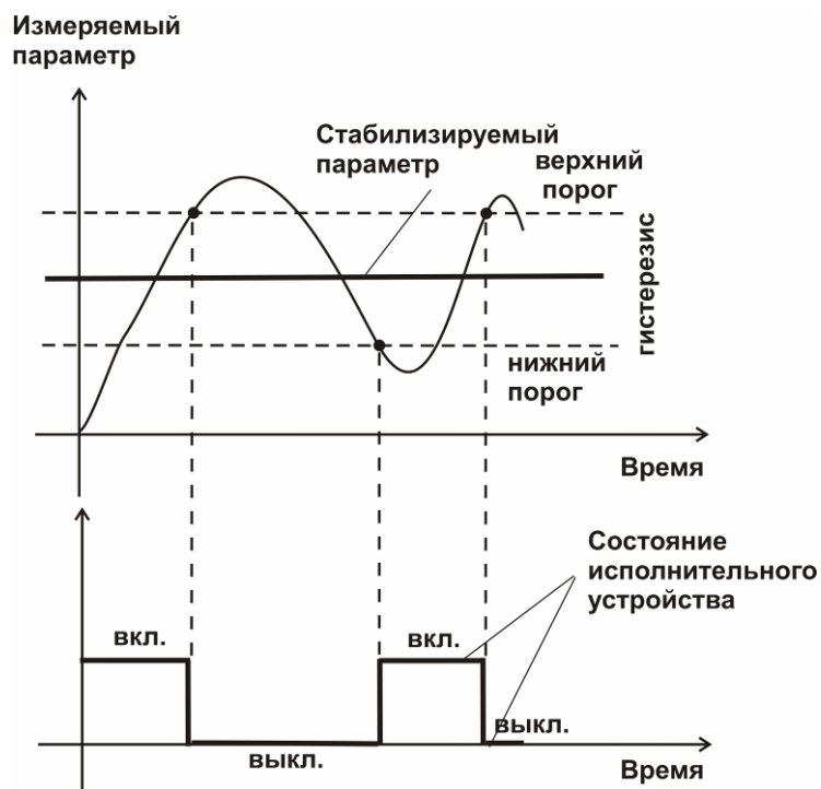
Рисунок 3.15 Стабилизация с гистерезисом (нагреватель)
