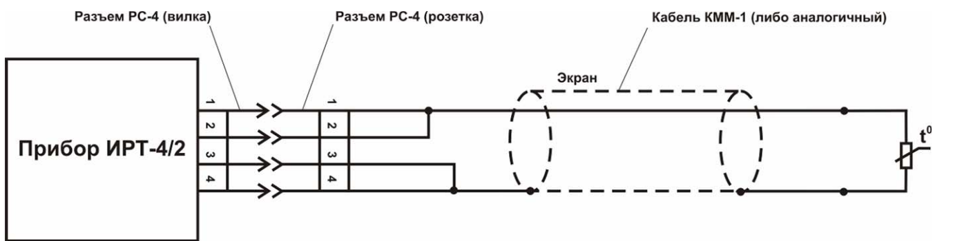
Рисунок 3.6 Двухпроводная схема подключения
