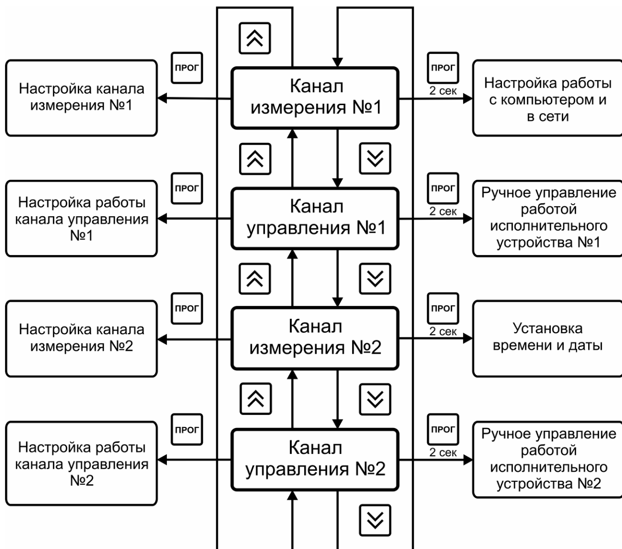
Рисунок 6.1 Режим РАБОТА
