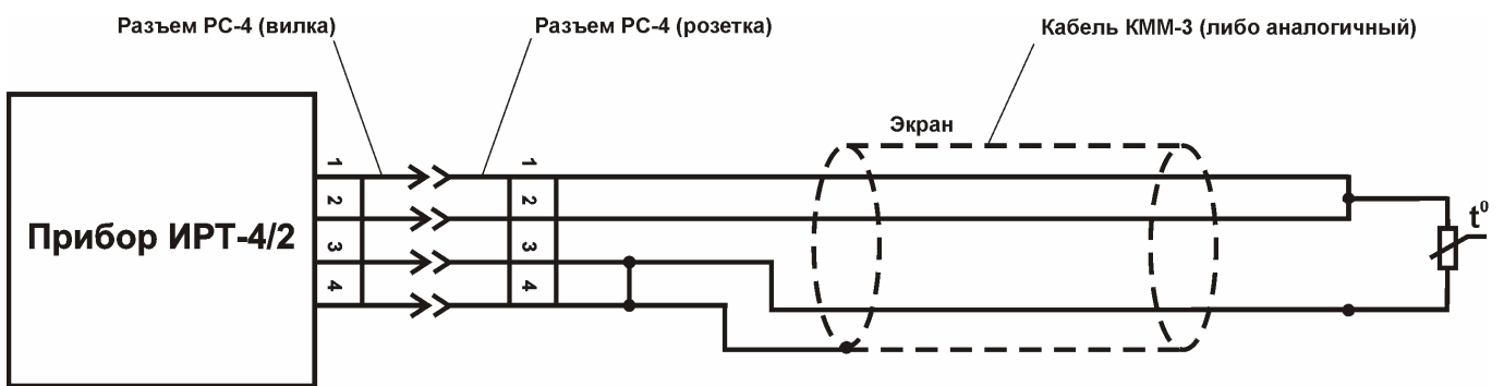
Рисунок 3.5 Трехпроводная схема подключения
