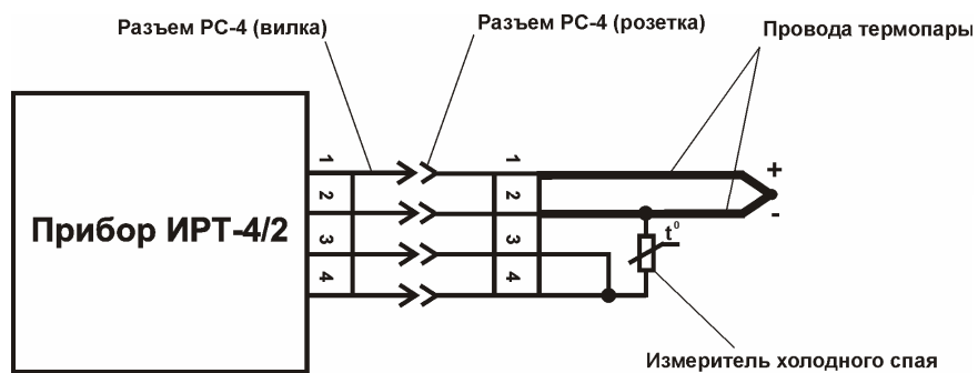
Рисунок 3.8 Схема подключения ТЭ преобразователей напрямую (без медных проводов) или удлиненных термоэлектродным кабелем
