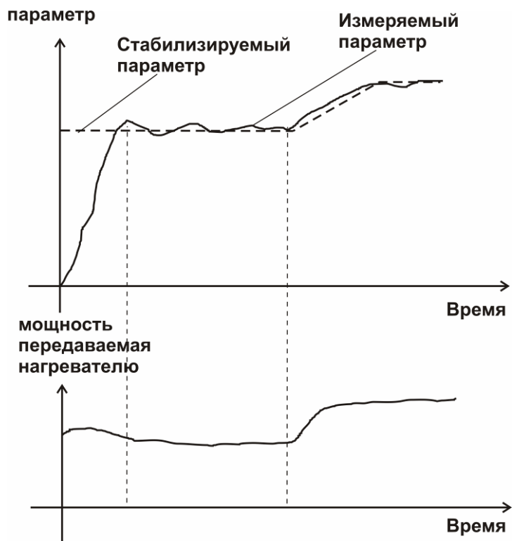
Рисунок 3.16 Стабилизация по ПИД закону (нагреватель)
