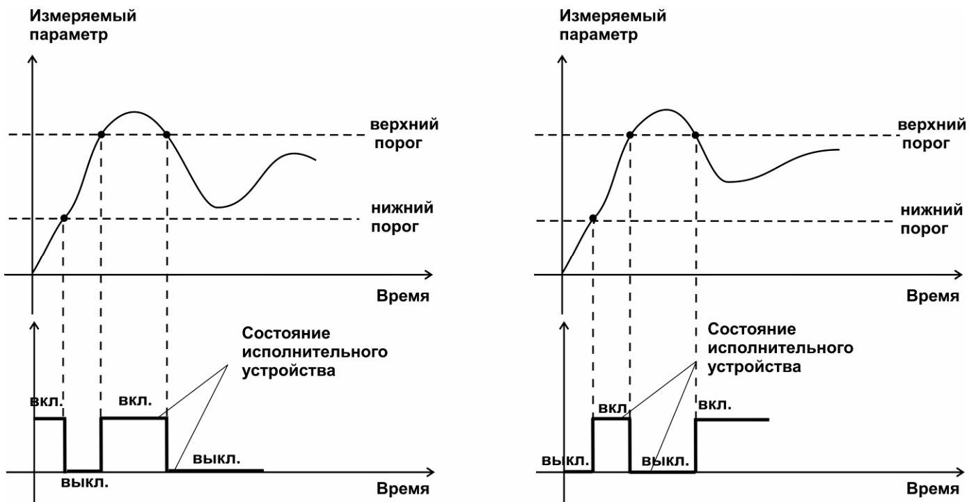
Рисунок 3.14 Функция вида f = НП+ВП , слева – сигнализация выхода измеряемого параметра за диапазон, справа – тоже с инверсией, сигнализация, что измеряемый параметр находится в диапазоне
