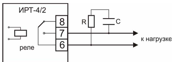
Рисунок 3.17 Подключение нагрузки к релейному выходу
