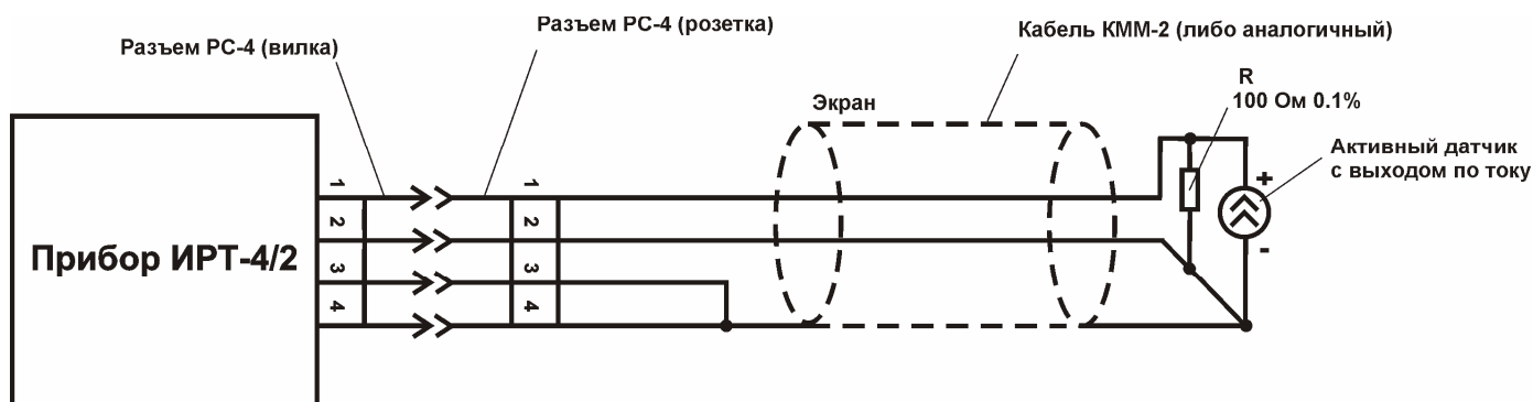
Рисунок 3.10 Схема подключения активного датчика с унифицированным токовым выходом (вариант 2)
