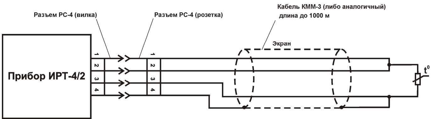
Рисунок 3.4 Четырехпроводная схема подключения
