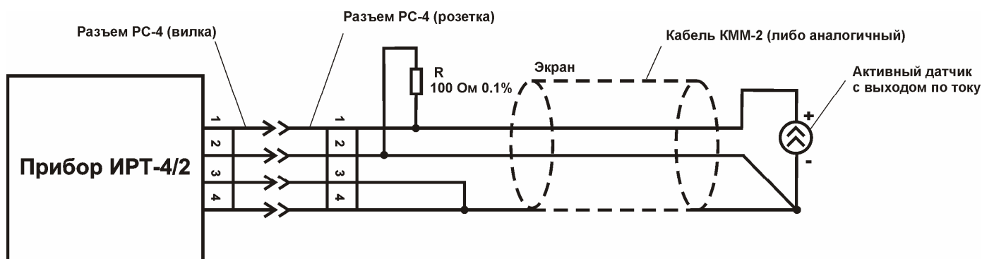
Рисунок 3.9 Схема подключения активного датчика с унифицированным токовым выходом (вариант 1)
