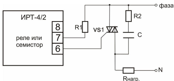
Рисунок 3.18 Схема подключения силового симистора
