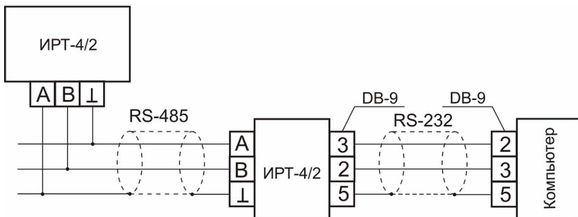
Рисунок 3.12 Использование функции преобразователя интерфейсов (позволяет избежать использования дополнительного преобразователя)
