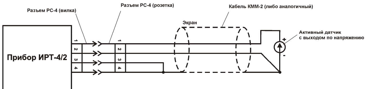
Рисунок 3.11 Схема подключения датчика с выходом по напряжению
