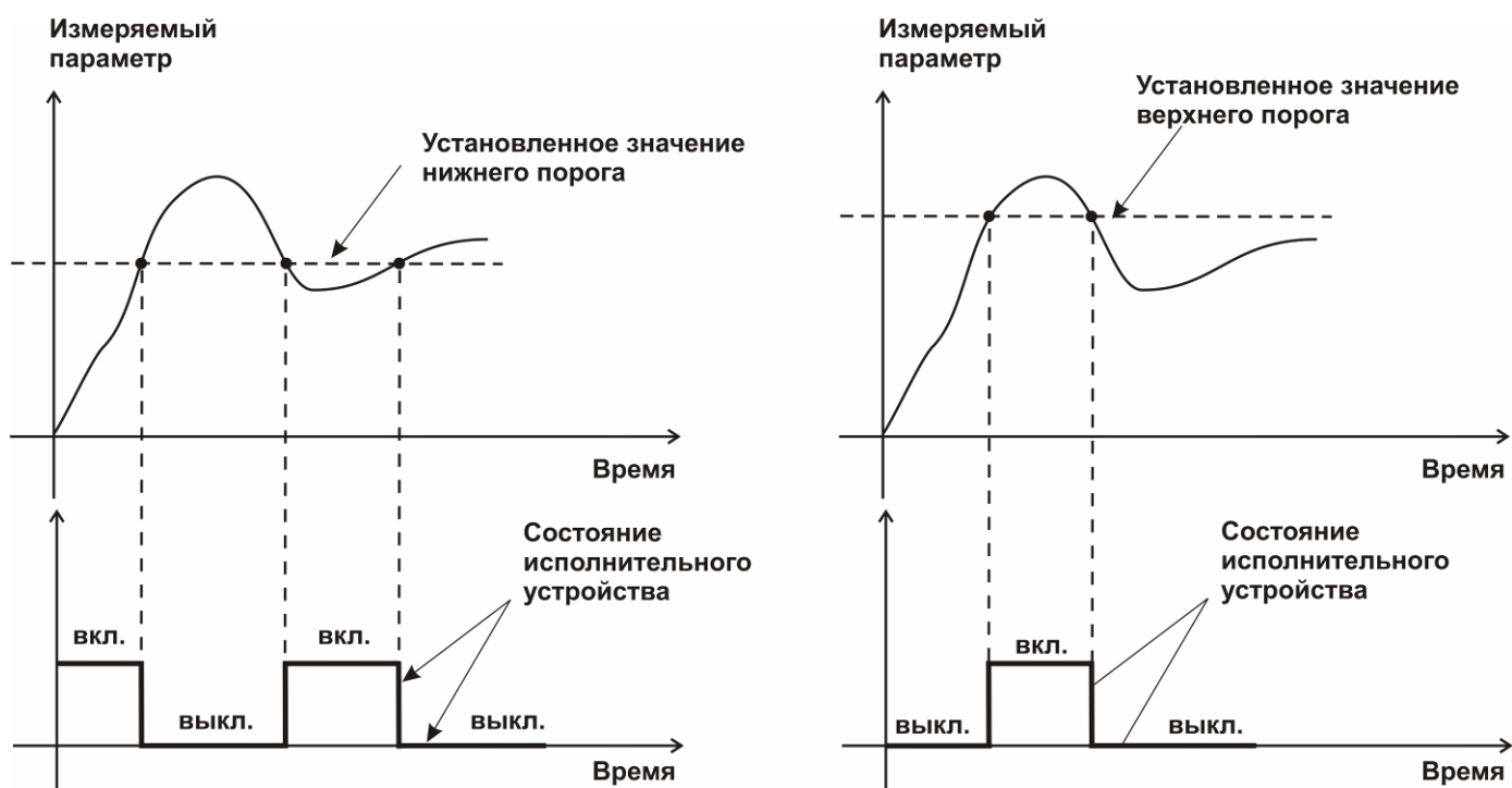
Рисунок 3.13 События: нарушения НП (слева), нарушение ВП (справа).
